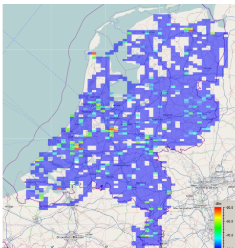
WiFi gebruik tussen 5470 en 5725 MHz in Nederland
